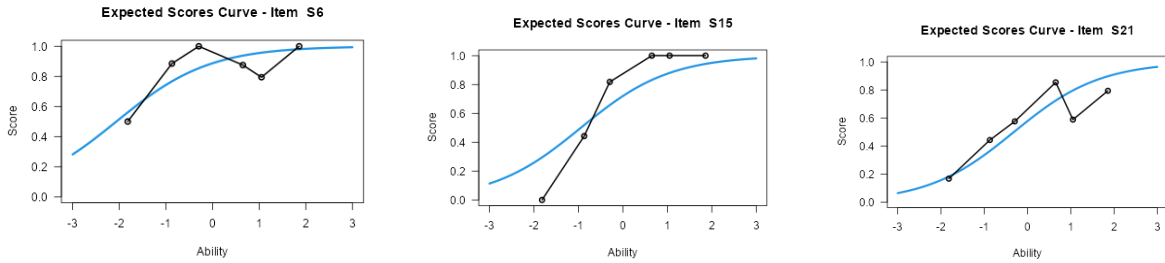
Görsel 1. Başarı testindeki S6 (En kolay madde), S15 (Ortalama güçlükte madde), S21 (En zor madde) maddelerine ilişkin karakteristik eğriler (MKE)
