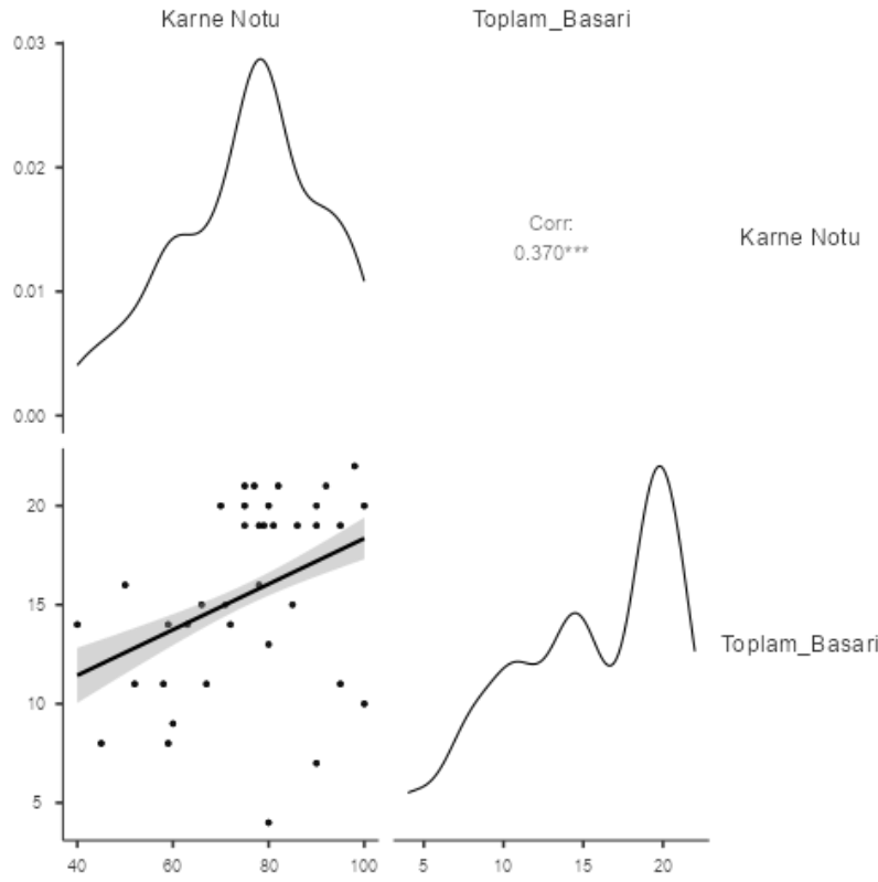
Görsel 3. Karne notu ile başarı puanı arasındaki ilişkiye ait saçılım grafiği ve yoğunluk eğrileri
